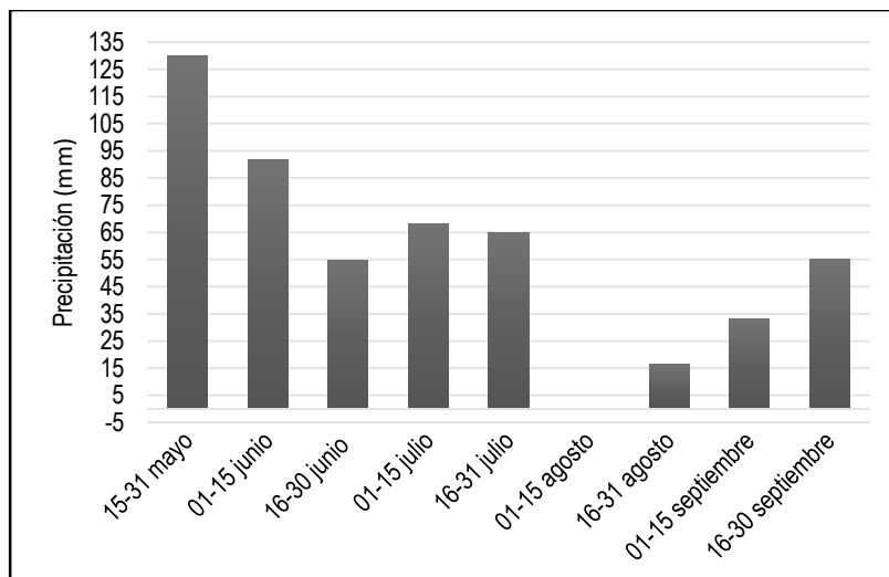
Figura 1. Distribución de la precipitación durante el ciclo agrícola primavera-verano 2025, en el CENID AF.
