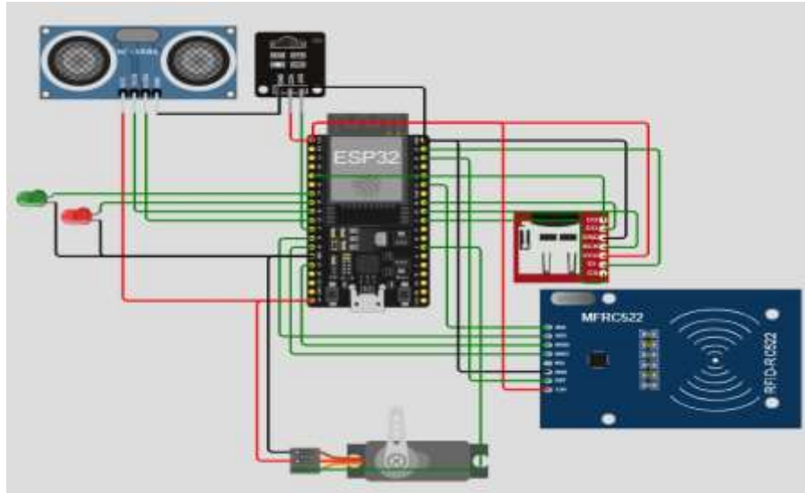
Figura 5. Maquetado de conexiones de sensores y actuadores al ESP32.
