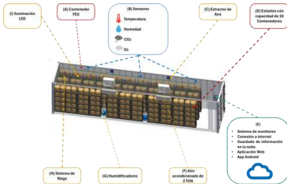
Figura 7. Modelado 3D de la cámara de morfogénesis fúngica.
