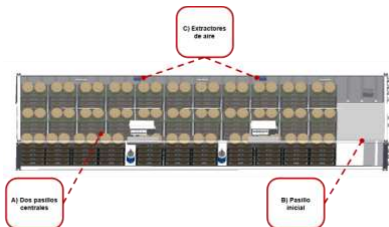
Figura 8. Distribución de la estantería de cultivo dentro de la cámara de morfogénesis fúngica.
