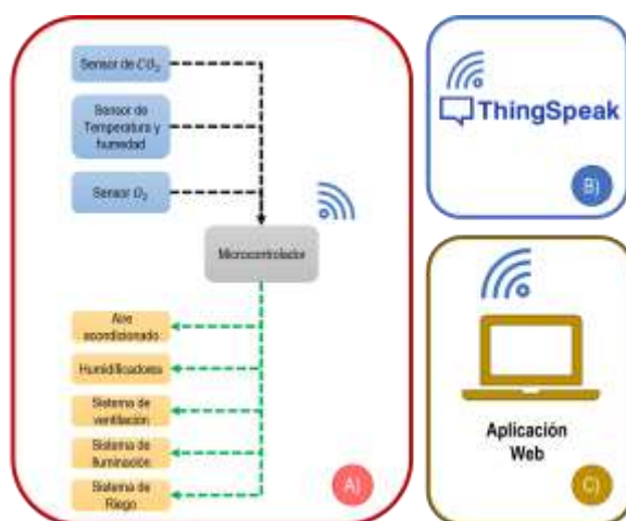
Figura 6. Arquitectura del sistema IoT propuesto: A) capa de percepción, B) capa de red, C) capa de aplicación
