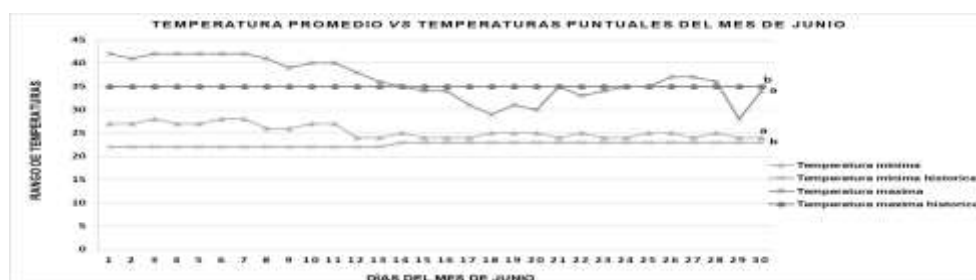
Figura 2. Valores promedios históricos diarios de temperaturas mínimas y máximas, valores temperatura diaria mínima y máxima, año 2024 mes de junio, fuente: Accuweather. Significancia, T de Wicolxon, p=0.00002 ; p=0.00005 < \alpha=0.005 , temperaturas máximas y mínimas en ese orden.
