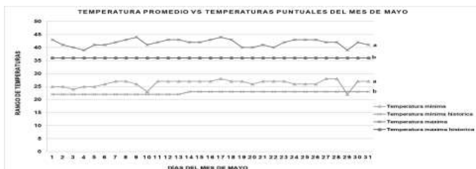
Figura 1. Valores promedios históricos diarios de temperaturas mínimas y máximas vs, valores temperatura diaria, mínima y máxima, año 2024 mes de mayo, fuente: Accuweather. Significancia, T de Wicolxon, p=0.00003 ; p=0.00002 < \alpha=0.005 , temperaturas máximas y mínimas en ese orden.
